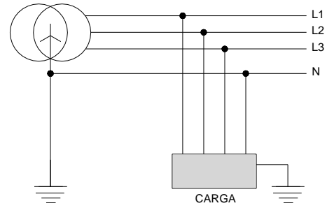
Figura 4 - Esquema TT
